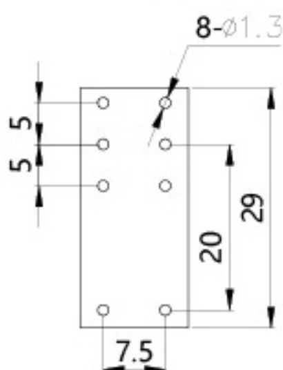
安装尺寸
