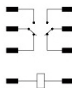
接线图
