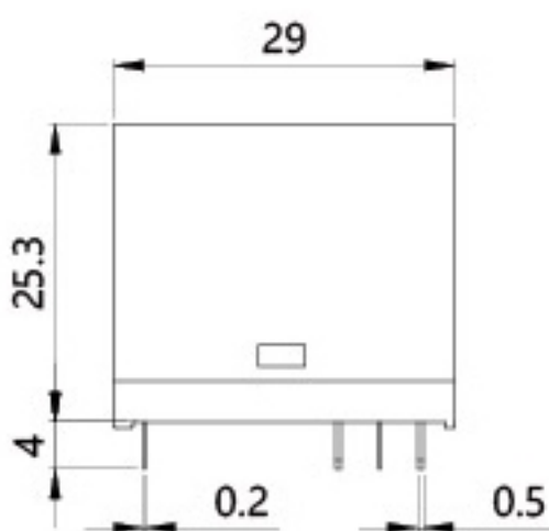
正面图
